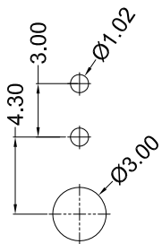
2P P.C.B LAYOUT
