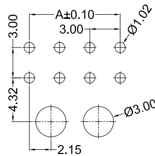
8P~24P P.C.B LAYOUT
