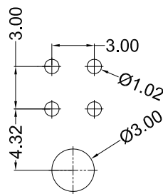
4P~6P P.C.B LAYOUT
